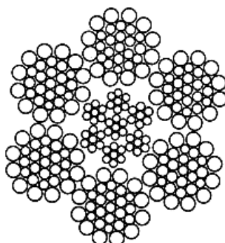
Шестипрядный канат 6х31+1 м. с.; 6х31=186 проволок с металлическим сердечником конструкции 7х7=49 проволок (прядь каната 1+6+6/6+12; прядь сердечника 1+6).
